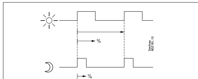
Rahmen-heizung
