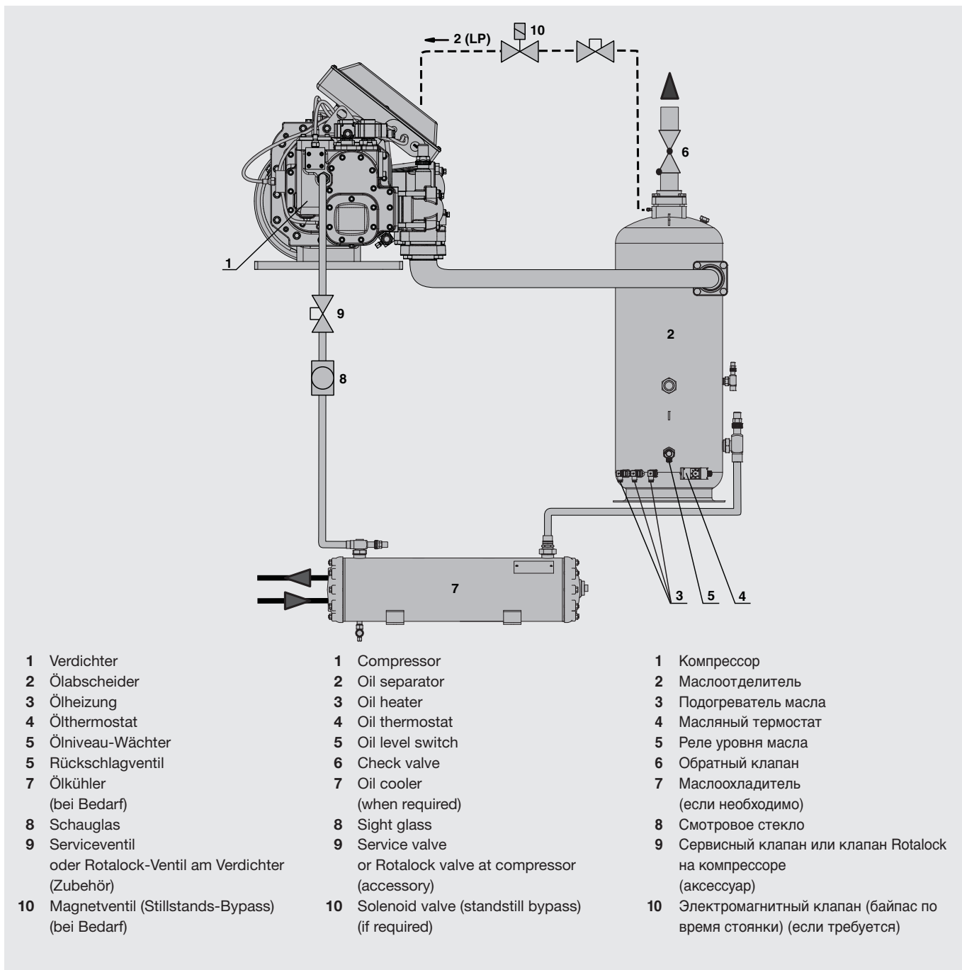
Abb. 8 Schmierölkreislauf
