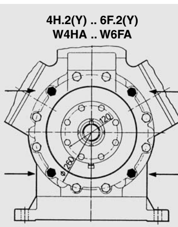
Fig. 5 Points de fixation pour la cage d'accouplement.
