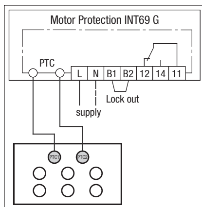
Рис. 21 Клеммная коробка
